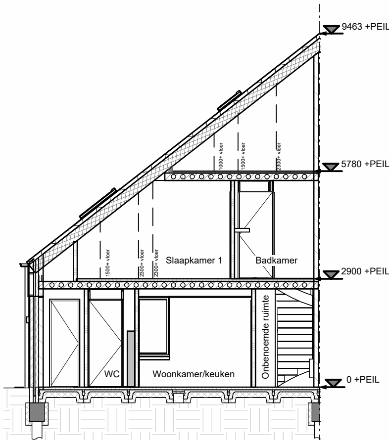
Doorsnede
