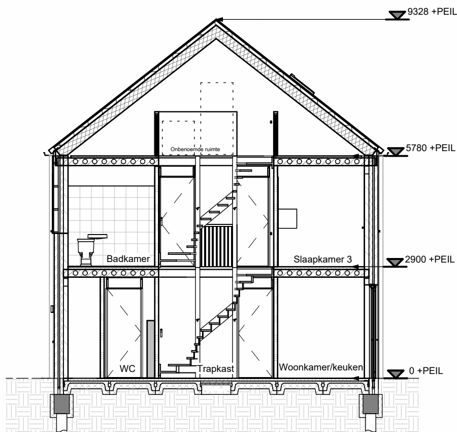
Doorsnede
